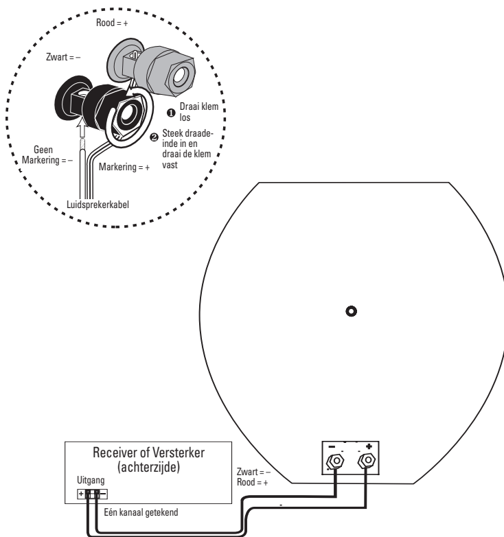
Afbeelding 3. Het blokschema geeft de juiste polariteit aan voor één kanaal van een home theater systeem.
